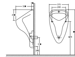
Urinoir (boveninlaat) Urinoir (orifice d'admission supérieur) Urinal (inlet above) (code S8600700000)
